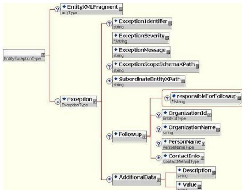
Figure 4 : Le type EntityExceptionType
