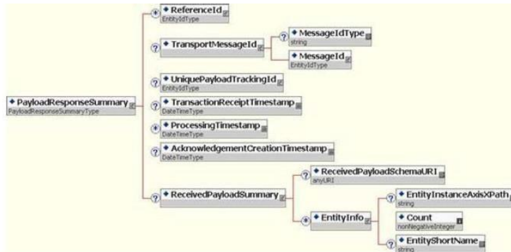
Figure 2 : Le type PayloadResponseSummaryType
